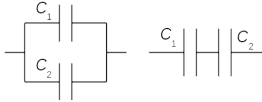
Рис. 3.4: Параллельное и последовательное соединение конденсаторов.
